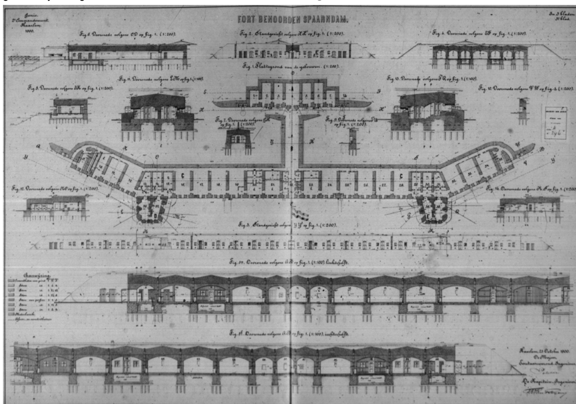
Plattegrond, doorsneden en standgezichten van gebouwen van het Fort benoorden Spaarndam. (NL-WpDStvA C8830, 1900)
