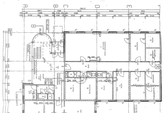
Plattegrond van een vleugel van gebouw T. (Jos Slats NL-WpDStvA-C8992, 1991)
